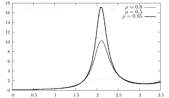
Graphe de \omega \mapsto \frac{1}{|1 + 2\rho e^{i\omega} + \rho^2 e^{2i\omega}|^2}
