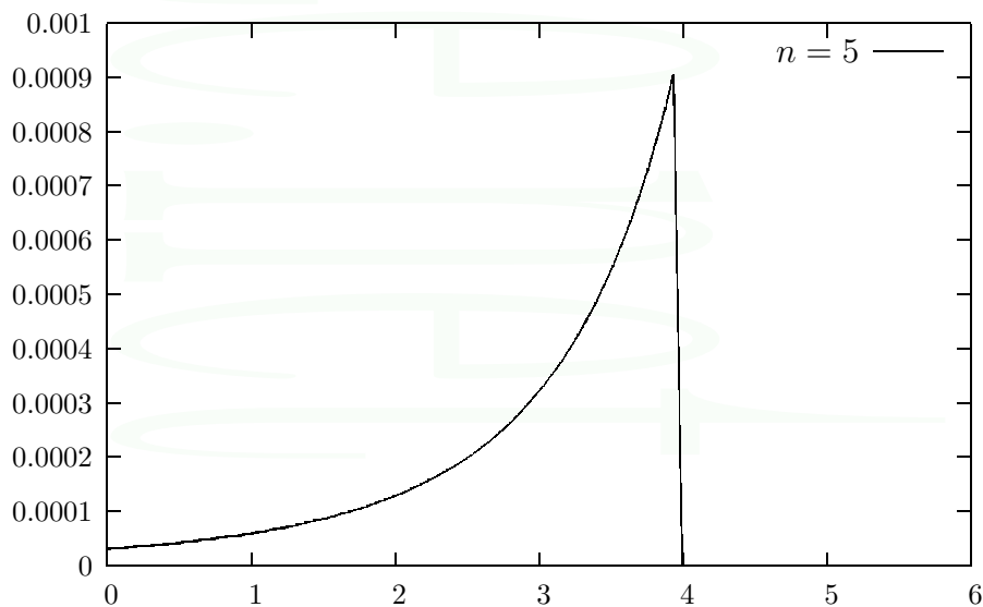
Graphique de a \mapsto L_X(x; a, b) lorsque b = 8 > \max_i x_i et \min_i x_i = 4
