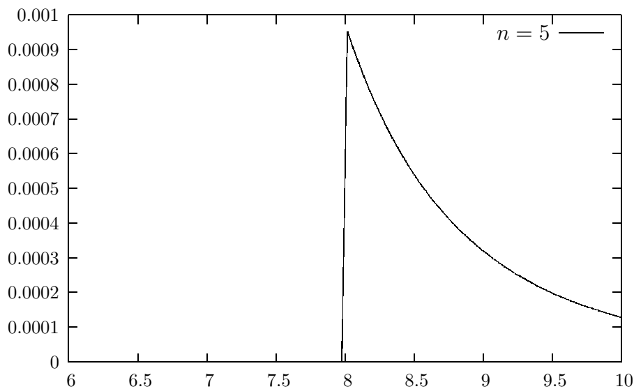
Graphique de b \mapsto L_X(x; a, b) lorsque a = 4 \leq \min_i x_i et \max_i x_i = 8
